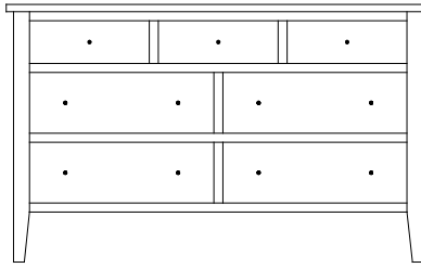
CS-1654 Dresser 59¼" w 36" h 21½" d w/7 drawers
